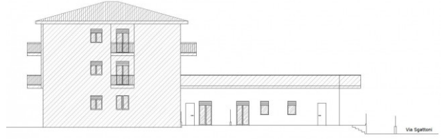
PROSPETTO OVEST
