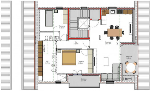
PIANTA PIANO SOTTOTETTO
