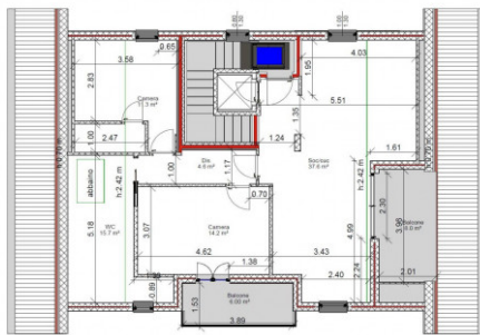
PIANTA PIANO SOTTOTETTO
