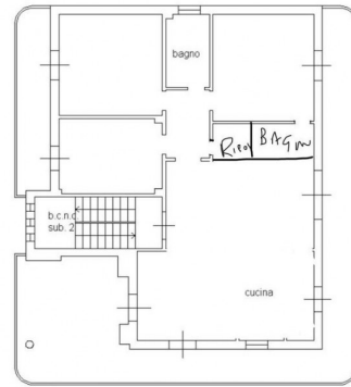
PIANTA PIANO PRIM h=2.85m
